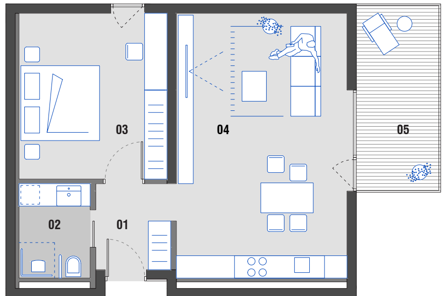
TLORIS STANOVANJA
