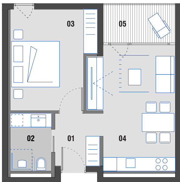
TLORIS STANOVANJA
