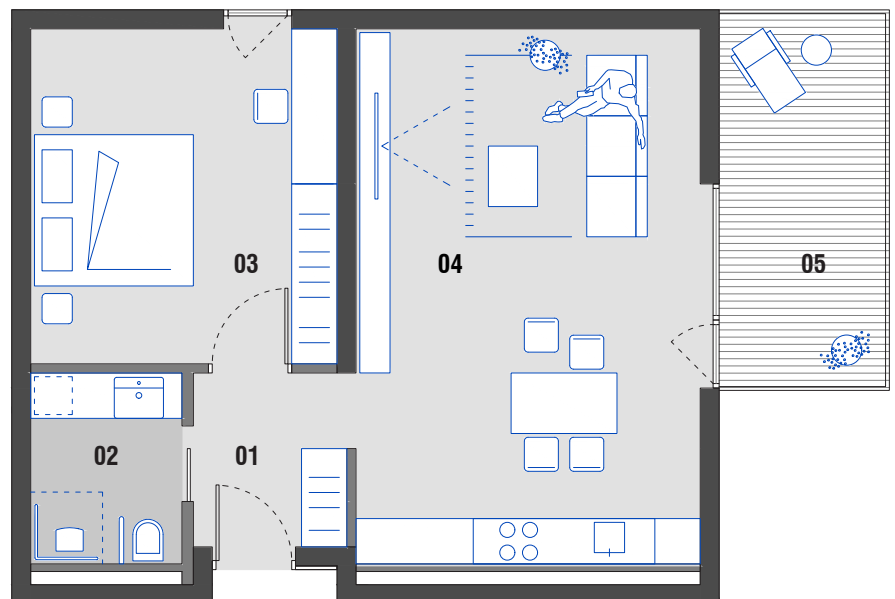
TLORIS STANOVANJA
